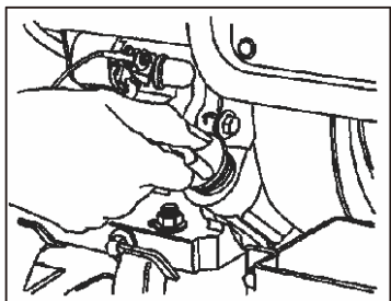
Рисунок 3. Проверка уровня моторного масла.
