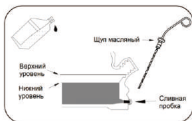
Рисунок 5. Отметки на масляном шупе.
