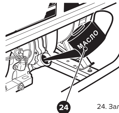
Рисунок 7 — Заливка масла в картер двигателя
