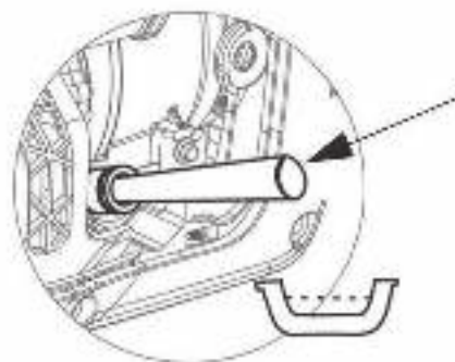
Рисунок 4-4. Отверстие для заливки масла с воронкой
