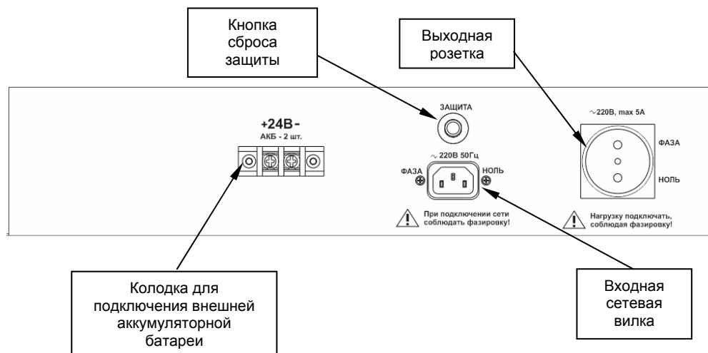
Рисунок 2 — Расположение разъемов для подключения.
