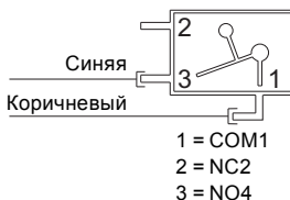
Рис. 1 Схема подключения
