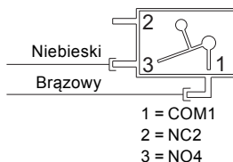
Rys. 1 Schemat połączeń
