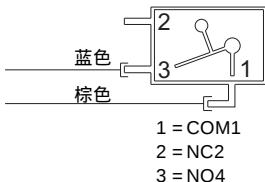
图 1 接线图
