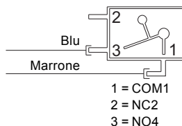
Fig. 1 Schema di cablaggio
