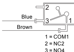
Fig. 1 Wiring diagram
