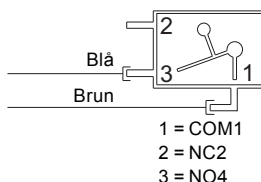
Fig. 1 Kopplingsschema
