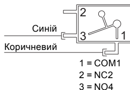
Рис. 1 Схема підключення
