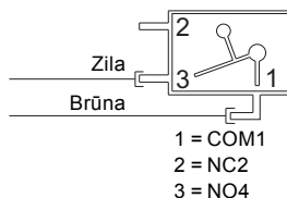
1. ilustr. Montāžas shēma
