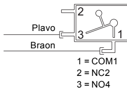
Slika 1 Dijagram ožičavanja
