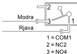
Slika 1 Shema ožičenja
