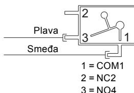
Slika 1 Dijagram ožičenja
