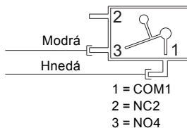
Obr. 1 Schéma zapojenia
