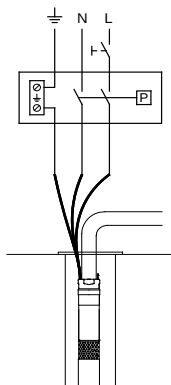
Tlakový spínač
