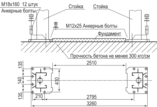
Рисунок 4 – Установочные размеры
