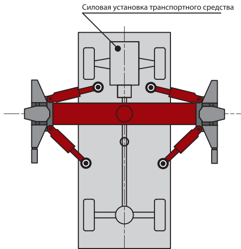
Рисунок 10 – Положение автомобиля
