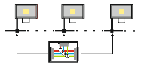
Рис. 1. Схема подключения прожектора к сети электропитания
