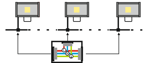
Рис. 1. Схема подключения прожектора к сети электропитания
