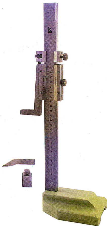
Рисунок 1 – Общий вид штангенрейсмасов торговой марки «Калиброн» с отсчетом по нониусу
