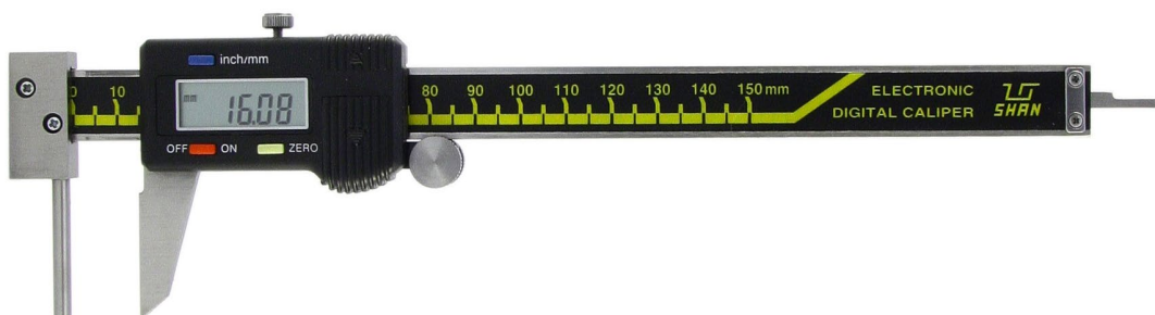
Рисунок 14 – Общий вид штангенциркулей модели ШЦЦСТ
