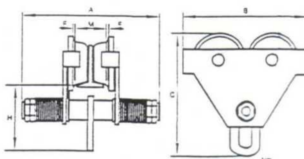
НЕПРИВОДНАЯ КОШКА
