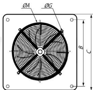
Компактный осевой вентилятор с защитной решеткой и монтажной панелью YWF B
