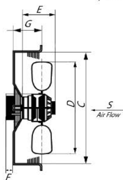
Компактный осевой вентилятор с защитной решеткой YWF S
