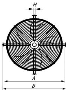
Компактный осевой вентилятор с защитной решеткой YWF S
