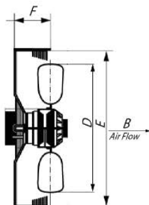
Компактный осевой вентилятор с защитной решеткой и монтажной панелью YWF B
