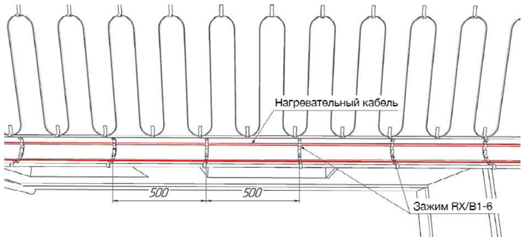
Рис. 3 (Зажим RX/B1-6)
