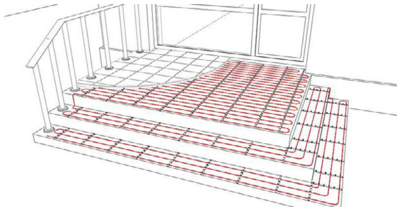
Рис. 3 (Вид сверху)
