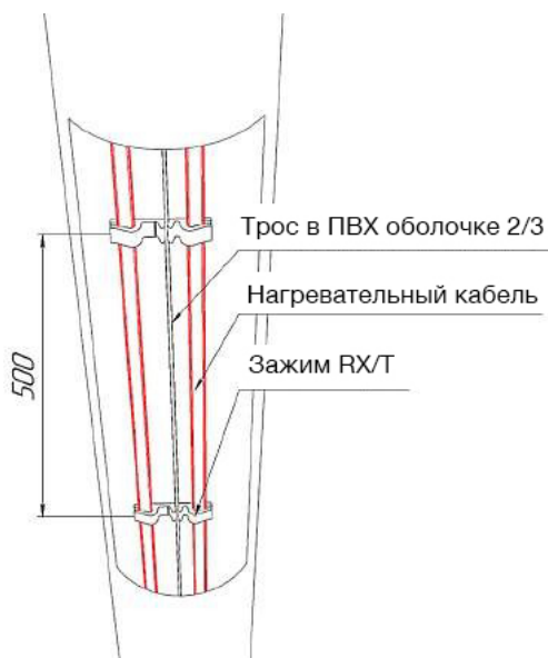
Рис. 5 (Зажим RX/Т)
