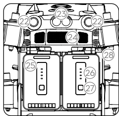
后视图
