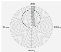
G-8 2.4GHz アンテナの方 位角平面パターン
