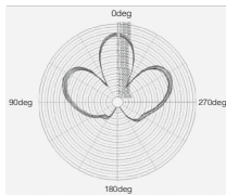
G-8 5.8 GHz アンテナ の方位角平面パターン
