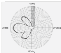
G-8 5.8 GHz アンテナ の仰角平面パターン
