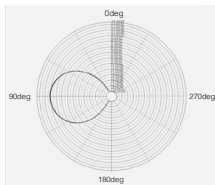
G-8 2.4GHz アンテナの 仰角平面パターン
