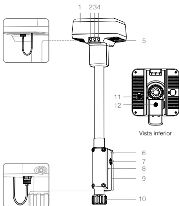
Cuerpo de la D-RTK 2
