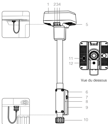
Boîtier de la D-RTK 2
