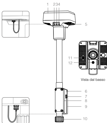
Corpo di D-RTK 2
