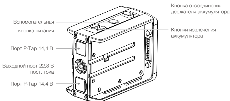
Двойное крепление аккумуляторов TB50
