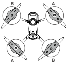
프로펠러와 모터 표시 매치하기
