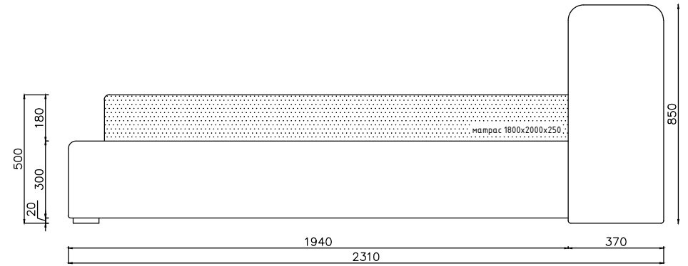
Вид сбоку
