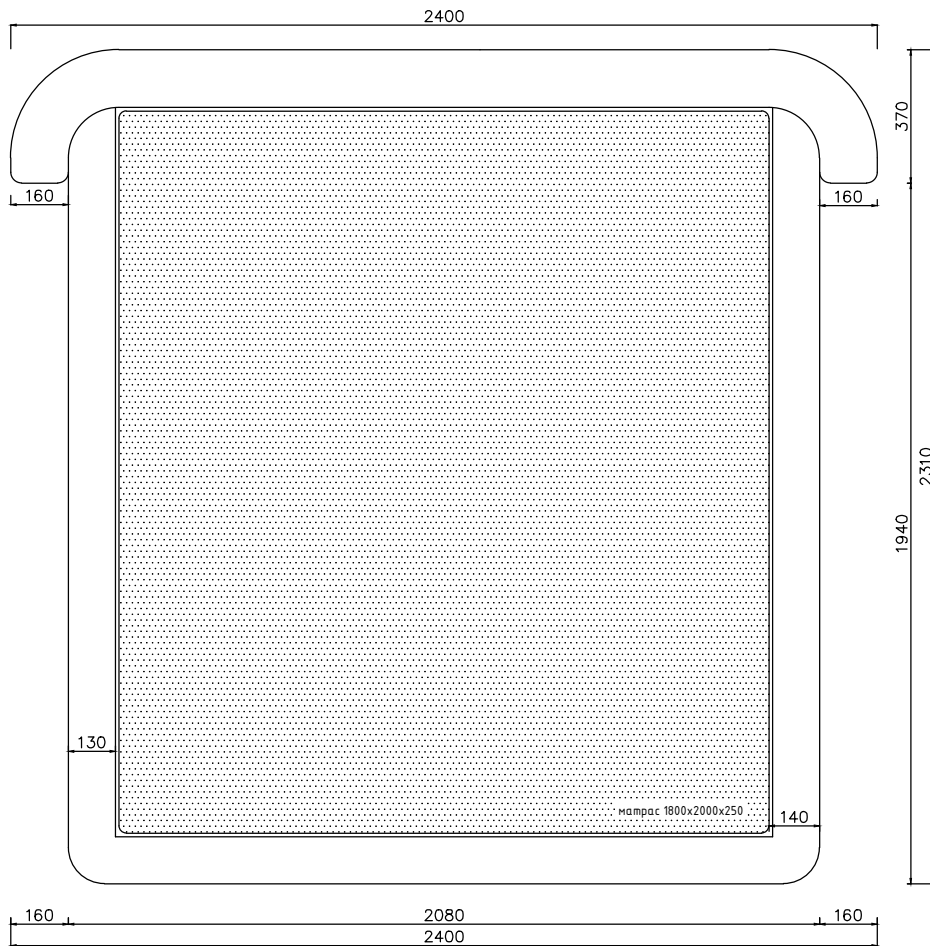
Вид сверху
