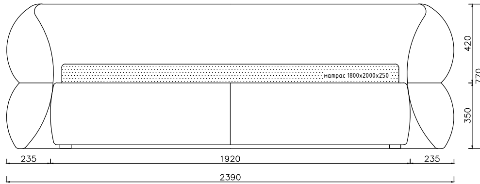
Вид спереди
