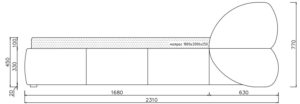
Вид сбоку
