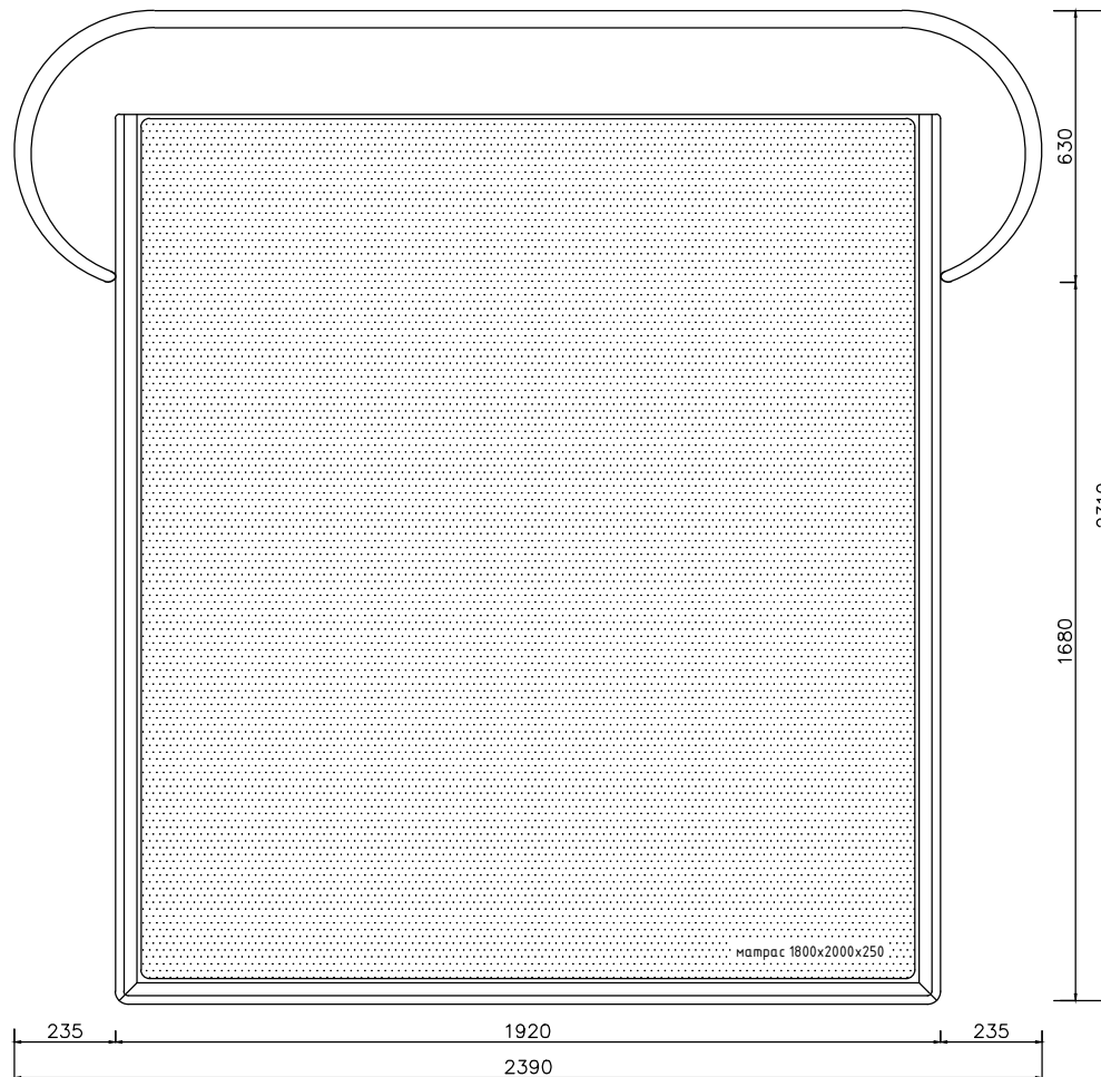
Вид сверху
