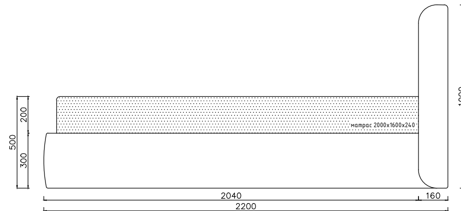
Вид сбоку
