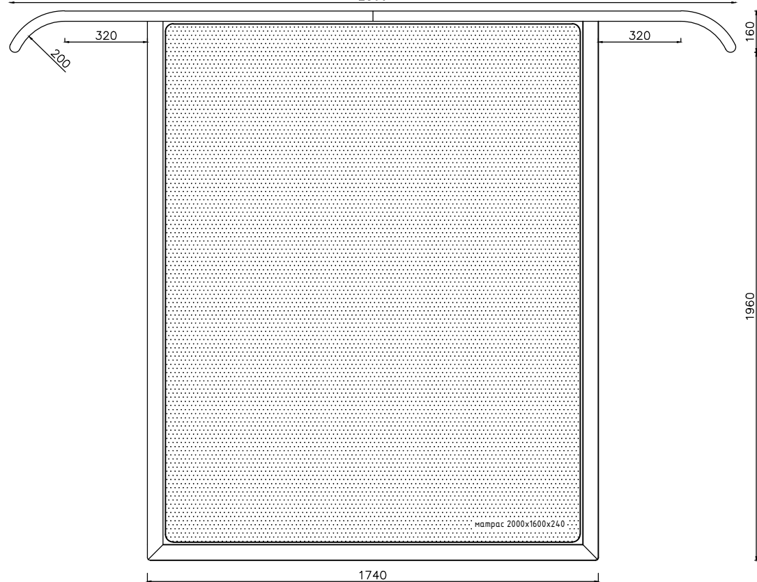
Вид сверху
