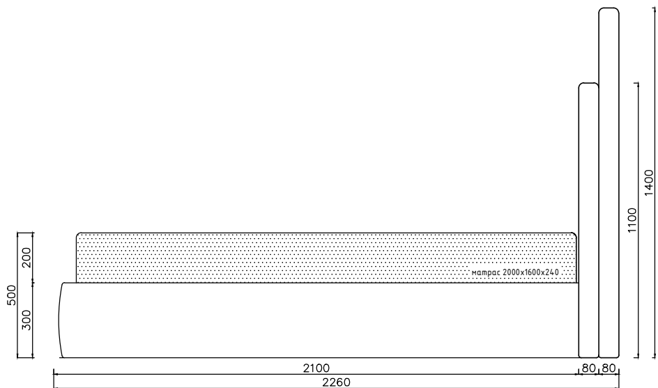
Вид сбоку
