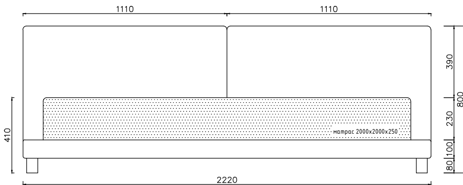
Вид спереди
