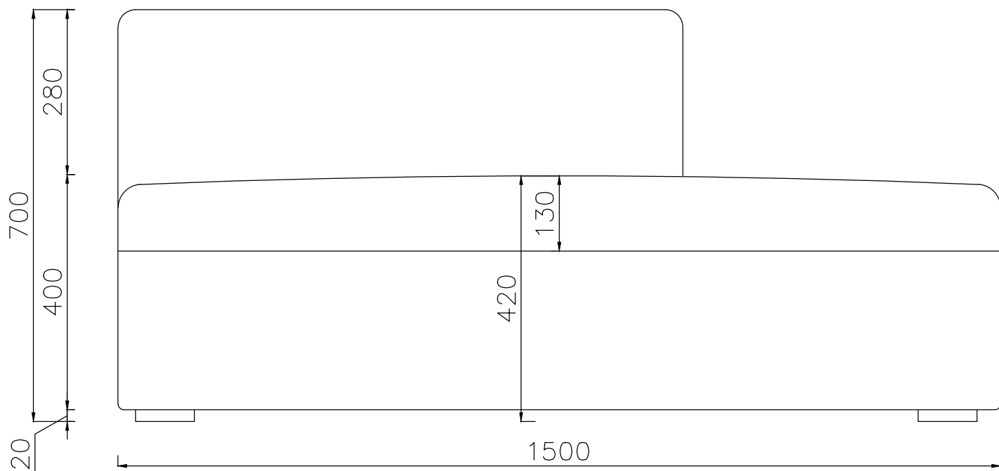
Вид спереди
