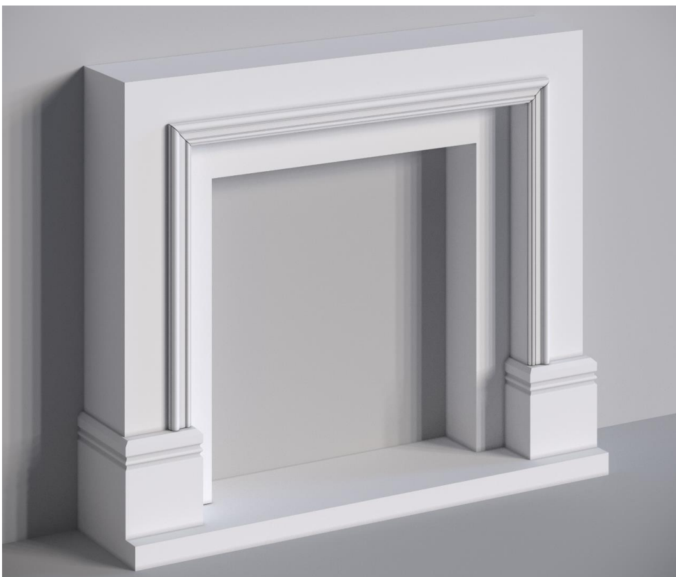
Рис. 6. Монтаж молдингов МО-1.076 (50 x 20 мм) на фронтальной части портала.
