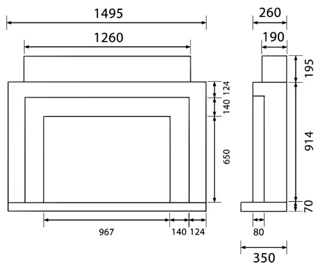
Рис. 1. Монтаж короба из ГКЛ с габаритами 1495 x 1179 x 350 мм.
