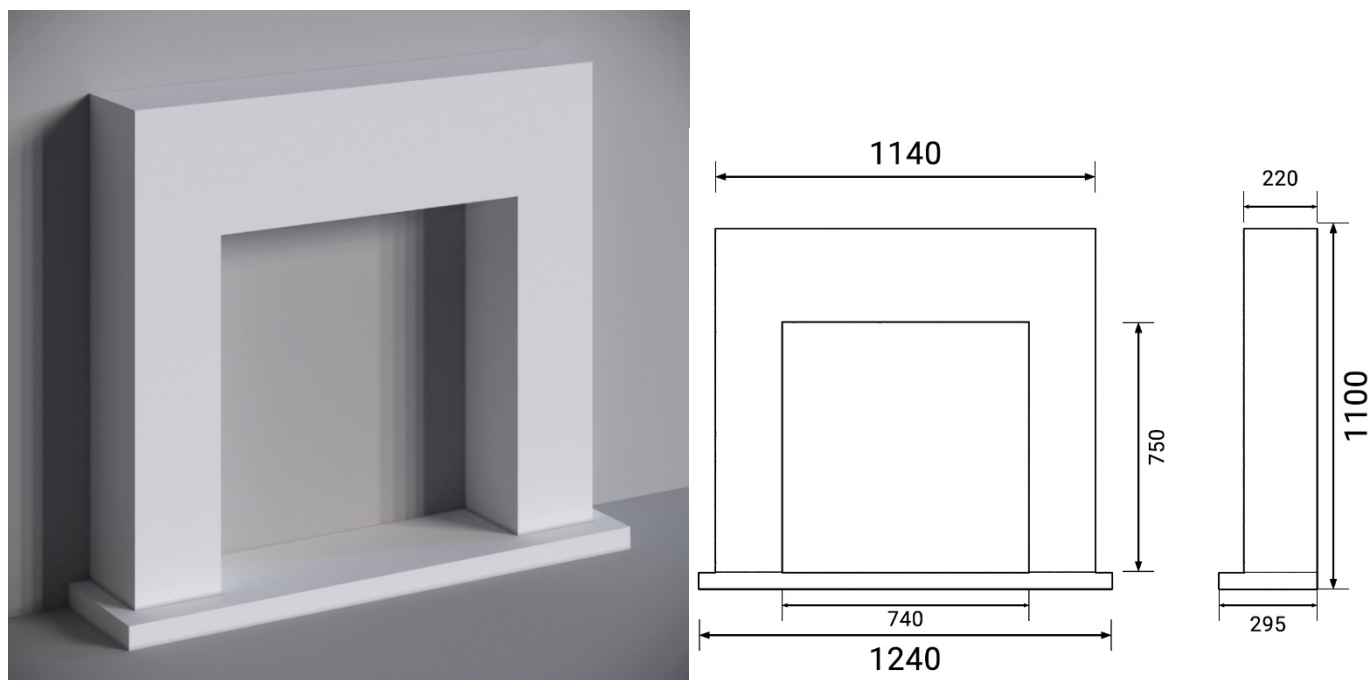
Рис. 1. Монтаж короба из ГКЛ с габаритами 1240 x 295 x 1100 мм.
