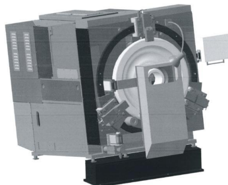
«Колесорасточной станок
