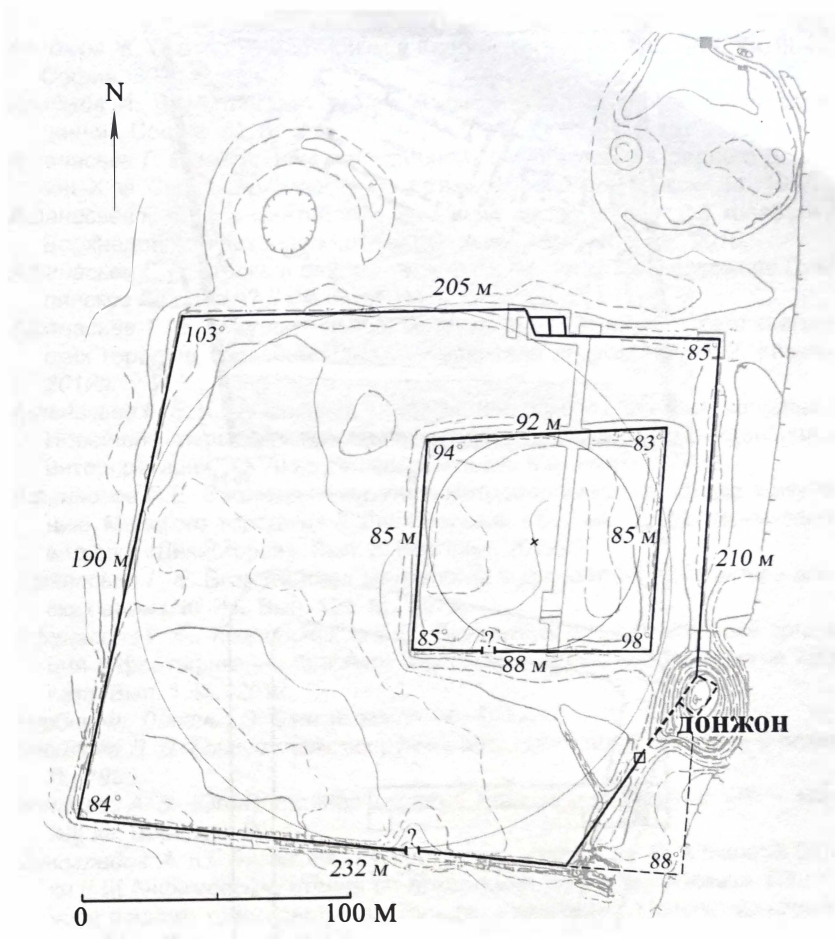
Илл. 5. Семикаракорская крепость. Вариант реконструкции В. С. Флёрова
