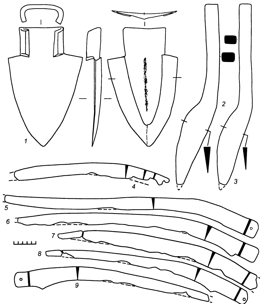
Рис. 5. Сельскохозяйственный инвентарь комплекса № 37
