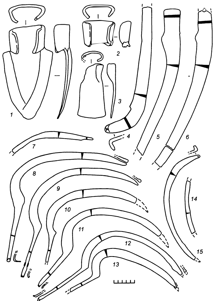
Рис. 3. Сельскохозяйственный инвентарь комплекса № 36
