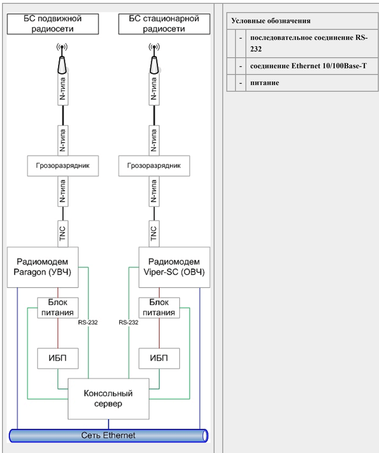
Рис. 1. Общая схема интегрированной БС АСОДУ ГТК «Иртыш»
