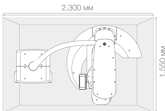
Вид сверху
