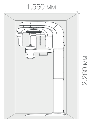
Вид сбоку
