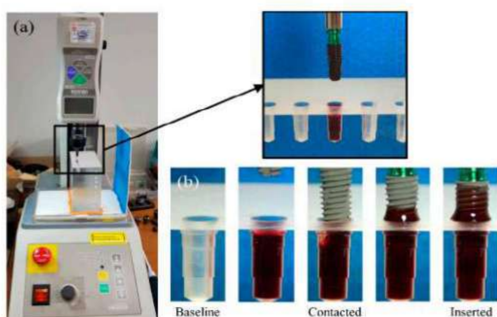
Рис. 2. Оценка динамической смачиваемости поверхности in vitro : (a) прозрачная акриловая пластина с отверстиями для имплантатов и силоизмерительное устройство; (b) исходная ситуация; апекс имплантата соприкоснулся с кровью; имплантат полностью ввели в отверстие
