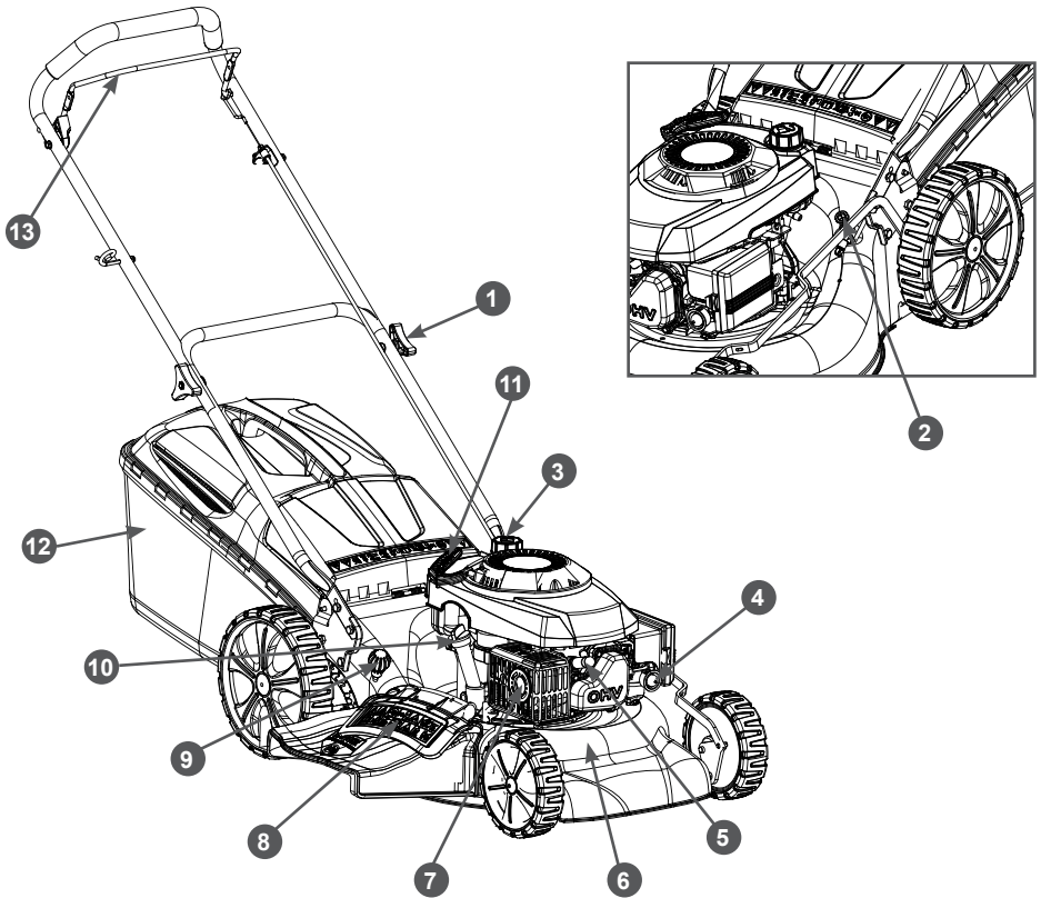
Рис. 1 Основные узлы и органы управления газонокосилки LM4622
